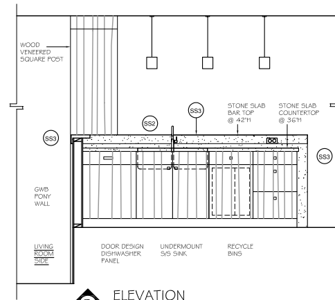
E ELEVATION
