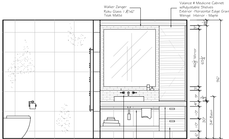
2 ELEVATION Scale: 1/4" = 1'-0"
